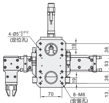
① 未使用安装组件时的安装图
