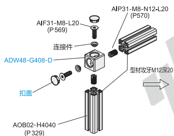
分解图
