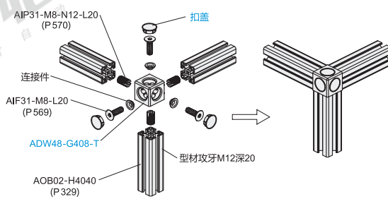
分解图
