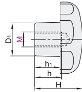
内螺纹型 HAU30 HAU33
