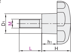
外螺纹型 HAU27 HAU28
