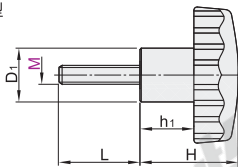
外螺纹型 HAU29
