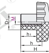
内螺纹型 HAU31 HAU32 HAU34
