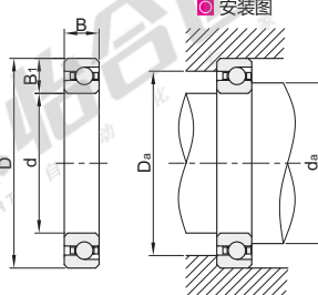
安装图
