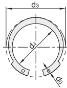
挡圈尺寸
