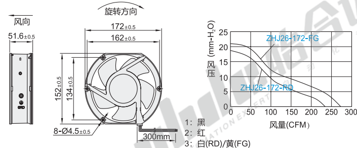
外形尺寸: 172
