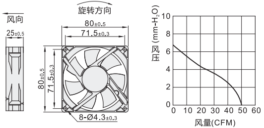
外形尺寸: 80
