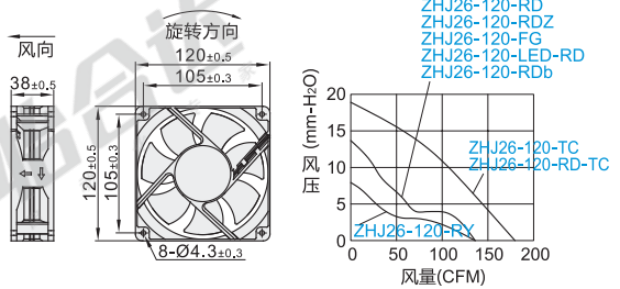
外形尺寸: 120
