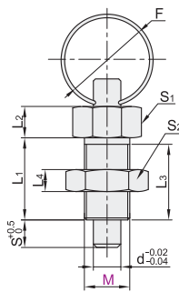
带锁紧螺帽 ZAC43 ZAC44 ZAC45
