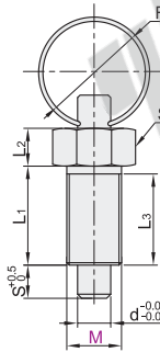
无锁紧螺帽 ZAC40 ZAC41 ZAC42
