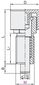
无锁紧螺帽 ZAB51 ZAB52
