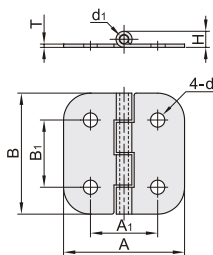
HFV16 4孔安装
