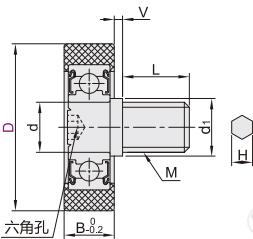
内六角外螺纹型 E-BKR22
