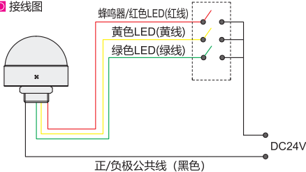
接线图
