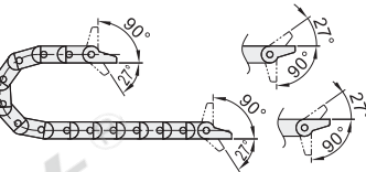
带销固定端(内部链节)
