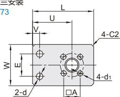
标准型·法兰安装 WIG71/72/73
