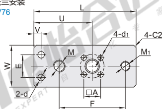
加宽型·法兰安装 WIG74/75/76
