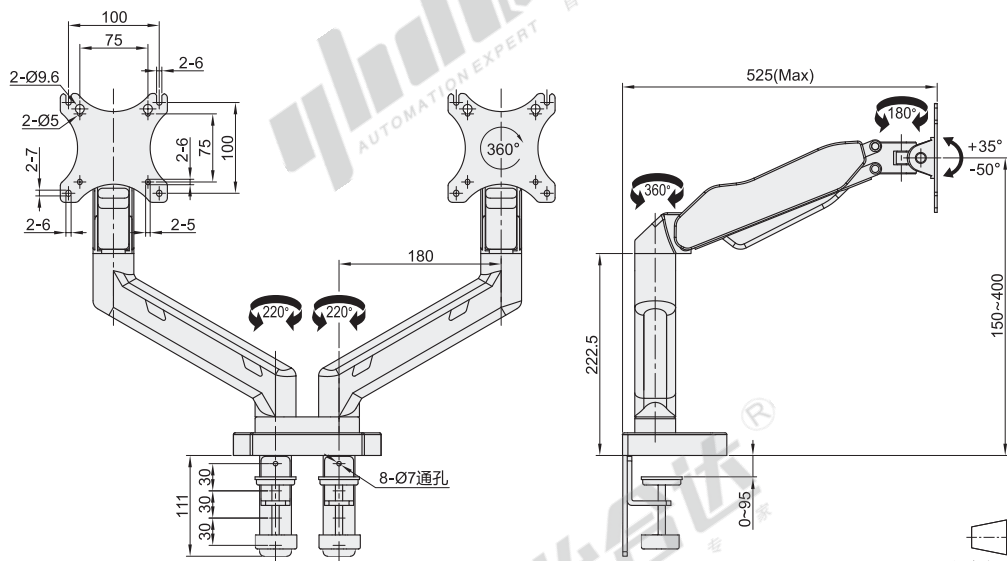
双显示器·四臂 NHD81
