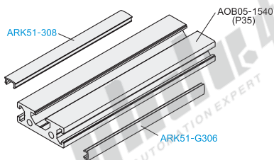
分解图
