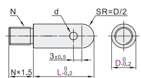
球头型 PAJ51/56
