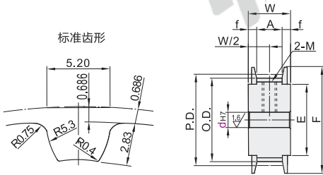
带轮形状：A形
