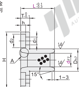
高强度黄铜合金 镶嵌固体润滑剂 E-OCR04
