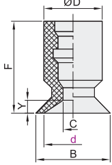
平形 盘径 \varnothing 2\sim 8
