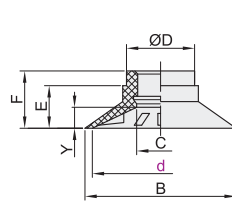
平形带肋 盘径 \varnothing 10\sim 32
