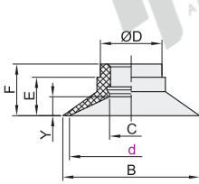
平形 盘径 \varnothing 10\sim 32
