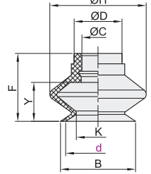
风琴形 盘径 \varnothing 10\sim 32
