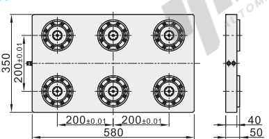
六中心零点卡盘 ZFH24 中心距:200
