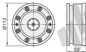
两中心零点卡盘 ZFH22 中心距:200
