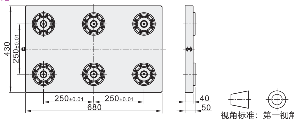
六中心零点卡盘 ZFH24 中心距:250
