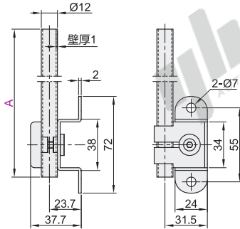
单管可调 ZLP55
