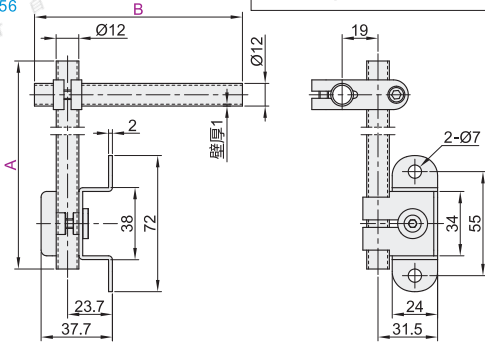
双管可调 ZLP56
