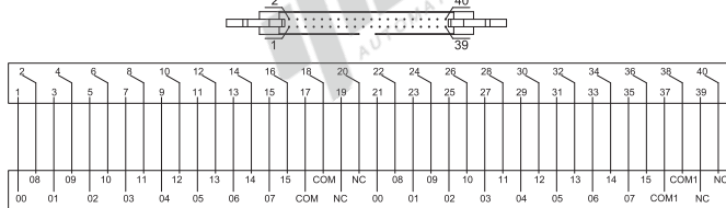
ZIU50-40A
