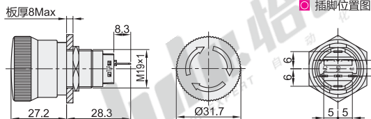
插脚位置图
