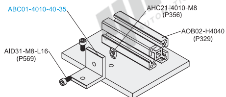
分解图
