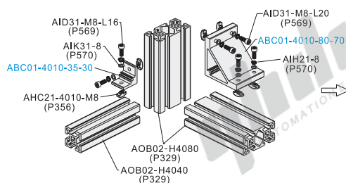
分解图
