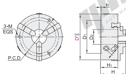
底部安装型 ZFH81
