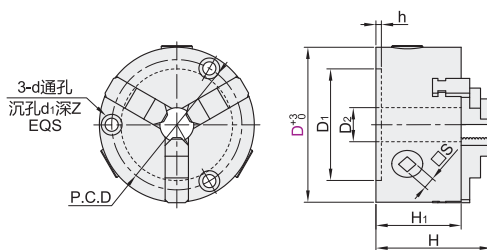
正面安装型 ZFH83
