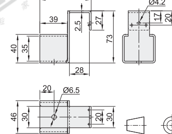
中间接头 QJK08
