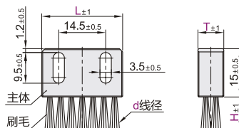
BMR56 (铝合金)
