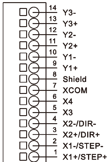
I/O连接器
