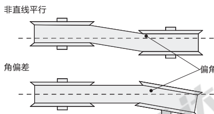
图1 皮带轮不对称图示
