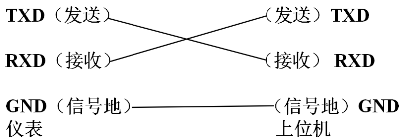
仪表与上位机接线图 (RS-232方式)
