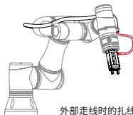
外部走线时的扎线固定
