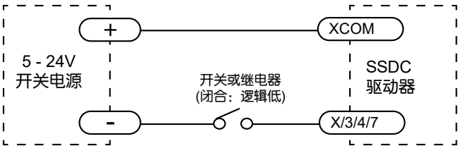
使用开关或继电器的连接方式
