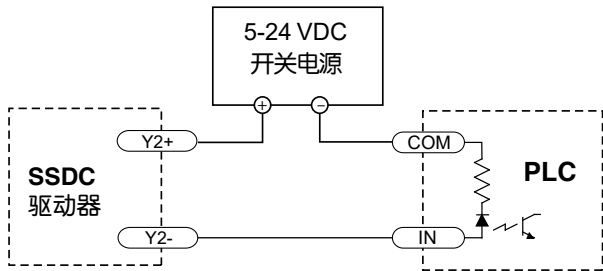
将输出Y2接成sourcing型输出，与PLC的输入相连
