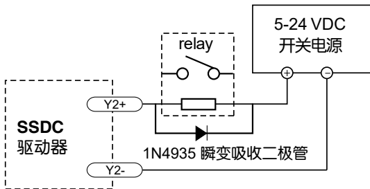
将输出Y2与继电器相连
