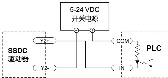
将输出Y2接成sinking型输出，与PLC的输入相连
