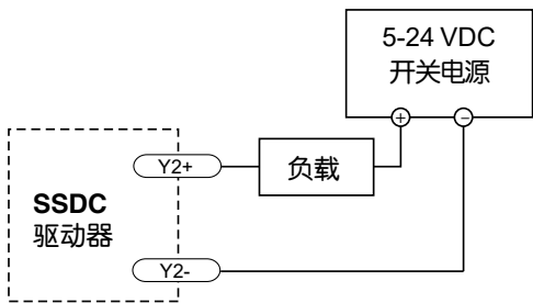
将输出Y2接成sinking型输出
