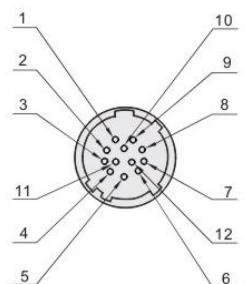
针排列图
