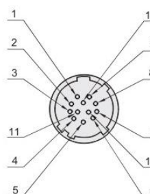
针排列图
