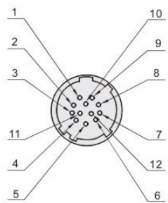
针排列图
