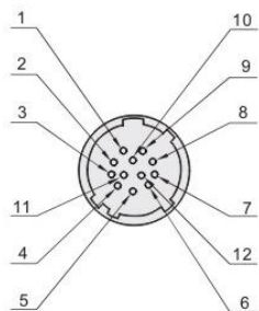
针排列图
