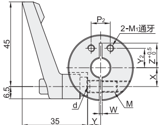
侧安装型 标准把手 FBM41/42/46
