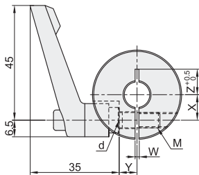
切割型 标准把手 FBM21/22/26
