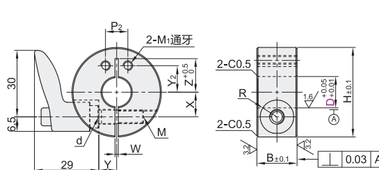
小型把手 FBM51/52/56
