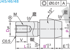
P.L.B.R尺寸指定型-圆型 YBU41/42/43 YBU45/46/48
