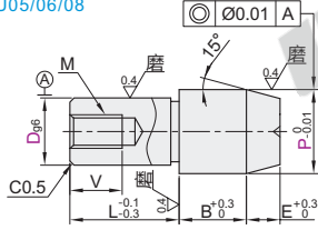
P.R尺寸选择型-圆型 YBU01/02/03 YBU05/06/08
