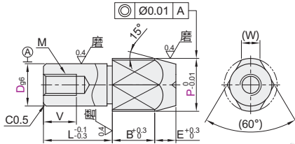
P.R尺寸选择型-多棱型 YBU11/12/13 YBU15/16/18
