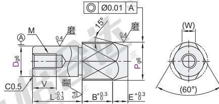
P.R尺寸选择型-多棱型 YBU20
