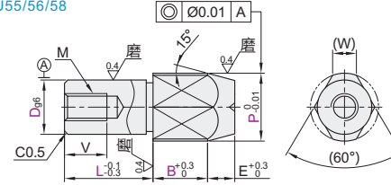
P.L.B.R尺寸指定型-多棱型 YBU51/52/53 YBU55/56/58
