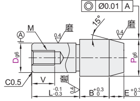
P.R尺寸选择型-圆型 YBU10
