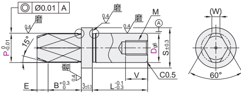
多棱型 YDR31/35
