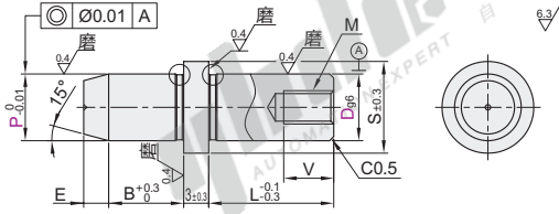
圆型 YDR21/25
