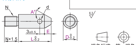
平头锥型 PAJ71/76
