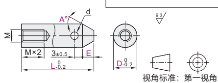
平头锥型 PAJ21/26
