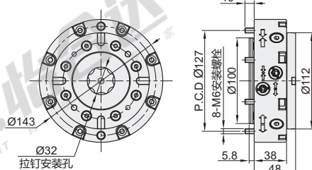
法兰型 ZFH54 带传感器
