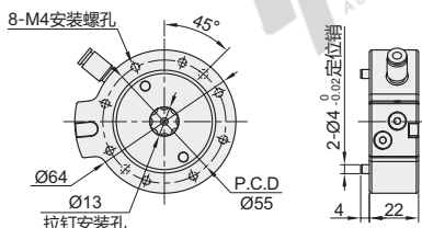
台面型 ZFH51 带传感器
