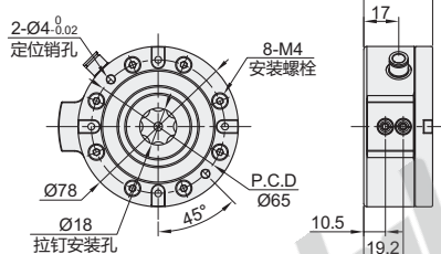
台面型 ZFH53 带传感器
