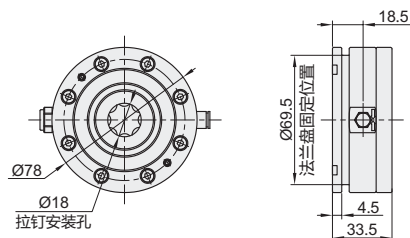
台面型 ZFH52 无传感器
