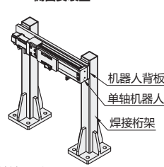
侧面安装型
