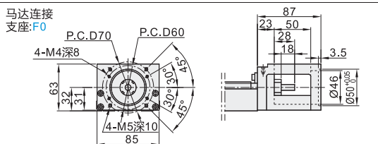
● 马达连接支座及与马达对应表
