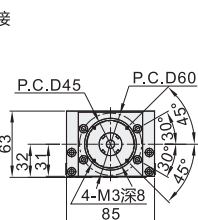
马达连接 支座:F3
