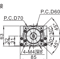
马达连接 支座:F1
