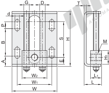
双弹簧调整型 ZCL63/64 W: 80
