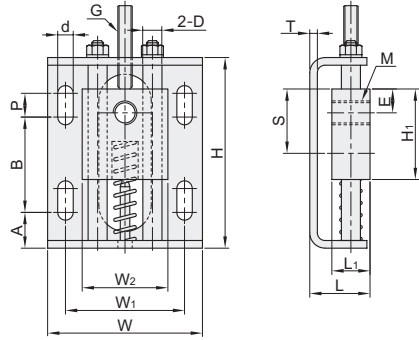
单弹簧调整型 ZCL62
