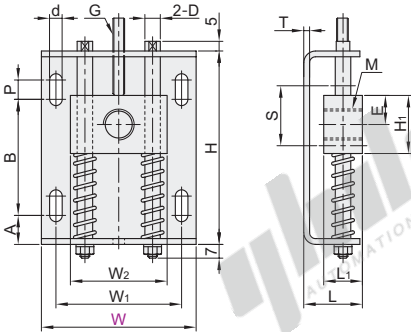
双弹簧调整型 ZCL63/64 W: 80
