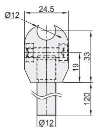
单圆管夹 ZCE03
