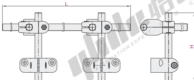
装夹组件+单圆管夹组合 ZCE55
