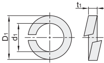
弹簧垫圈
