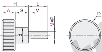
带台阶型-外螺纹型 PACK-TAR90/91/92/93
