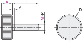
无台阶型-外螺纹型 PACK-TAR80/81/82/83
