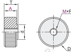
无台阶型-内螺纹型 PACK-TAR85/86/87
