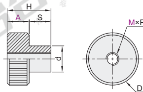
带台阶型-内螺纹型 PACK-TAR95/96/97
