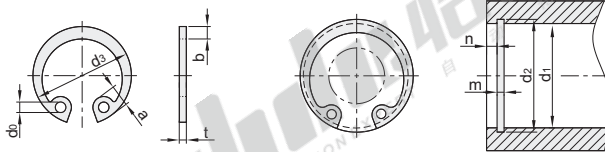
挡圈尺寸
