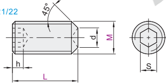
■ 平端(ML40Cr)
