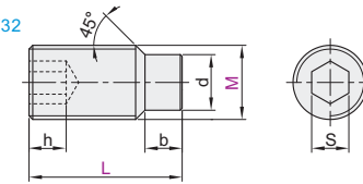
■ 锥端(ML40Cr)
