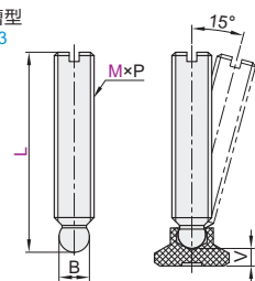
内六角孔型 TBD34
