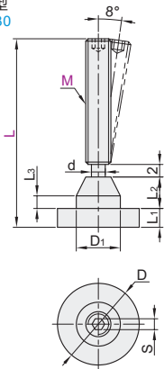
橡胶底座型 TBD31
