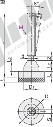
法兰底座型 TBD32
