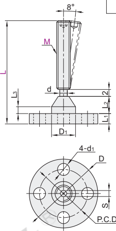
法兰底座型 TBD32
