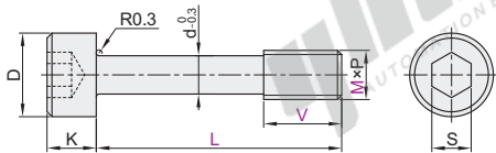
内六角圆柱头型 TBH32
