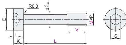
内六角短头型 TBH33
